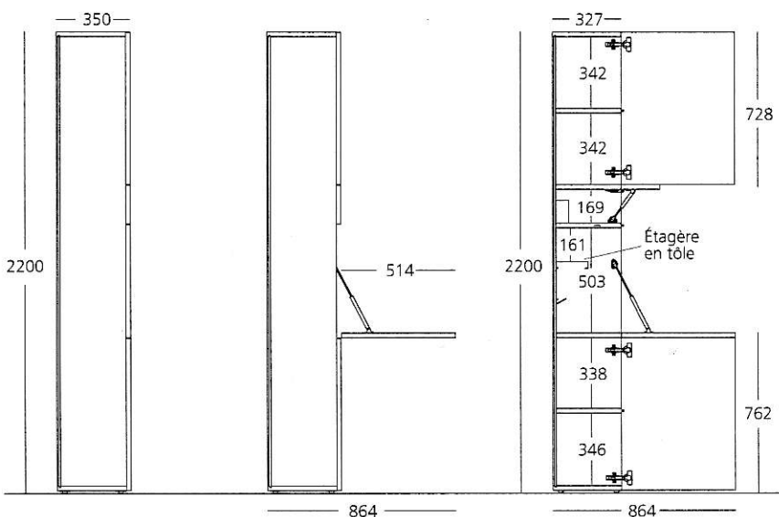
Meuble bureau fermé
