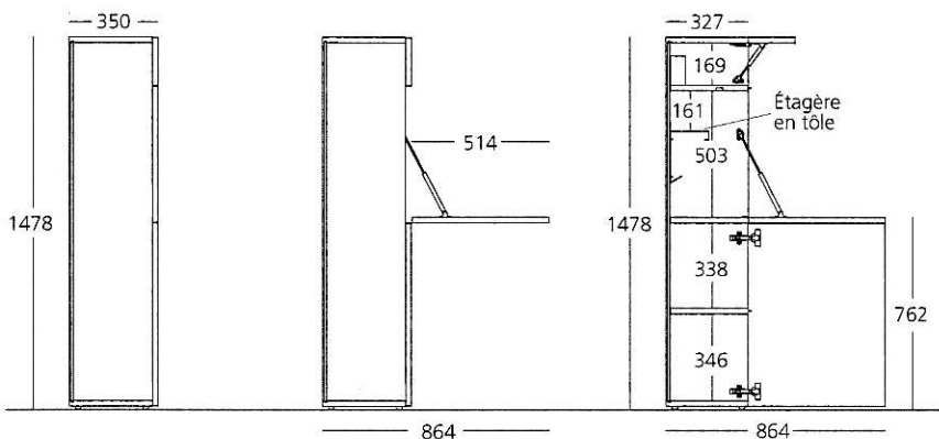
Meuble bureau fermé
