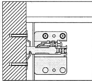
Détail de la fixation au mur en coupe
