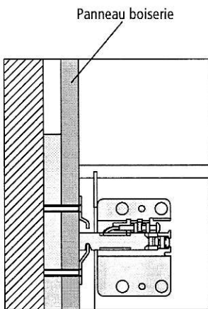
Détail de la fixation au panneau de boiserie
