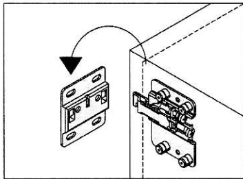
Détail du système de fixation au mur
